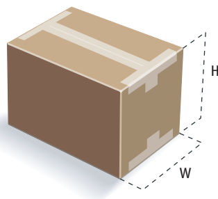
ההיקף מוגדר על פי הנוסחה: (2 \times \text{רוחב}) + (2 \times \text{גובה}) .
